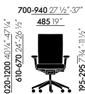
ID Soft L mit 3D-Armlehnen und Kleiderbügel
