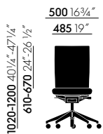
ID Soft L ohne Armlehnen
